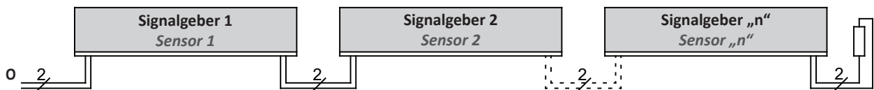
Bild 6: Verschaltung mehrerer Signalgeber, hier am Beispiel Sicherheitskontaktleiste
